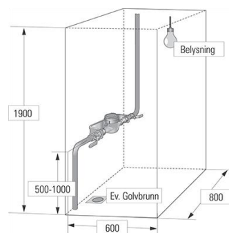
1. Skiss över installation med mätare och konsol.
